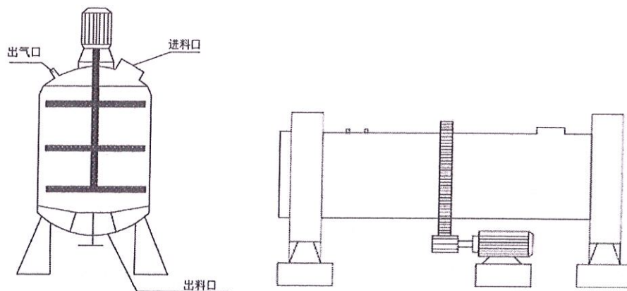
图 A.2-4 反应器式堆肥示意图（左为立式、右为卧式）
