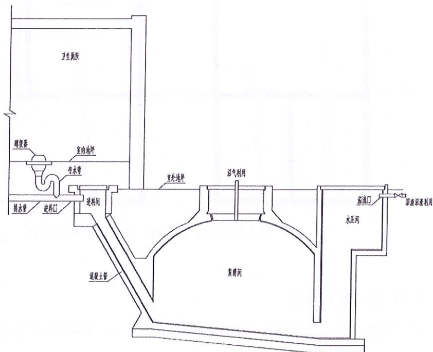
图 5.4-1 户厕沼气池示意图
