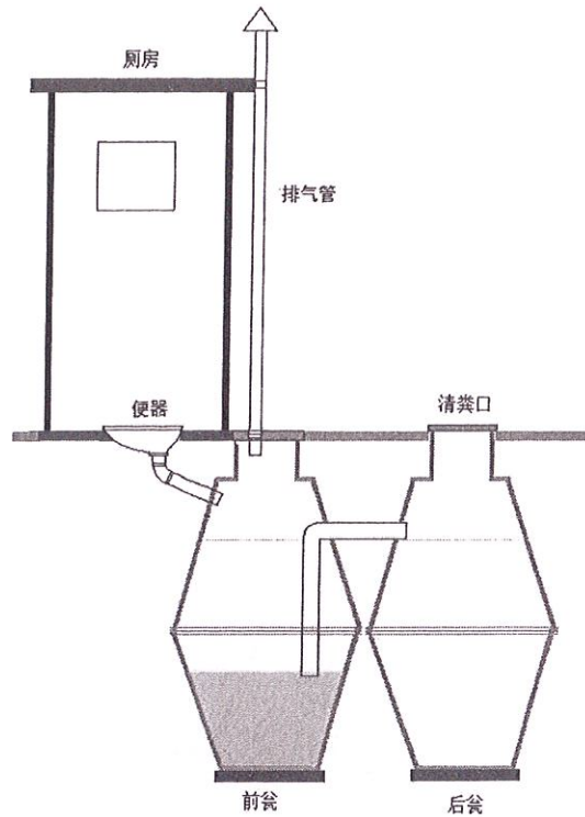
图 5.6-1 双瓮式户厕结构示意图
