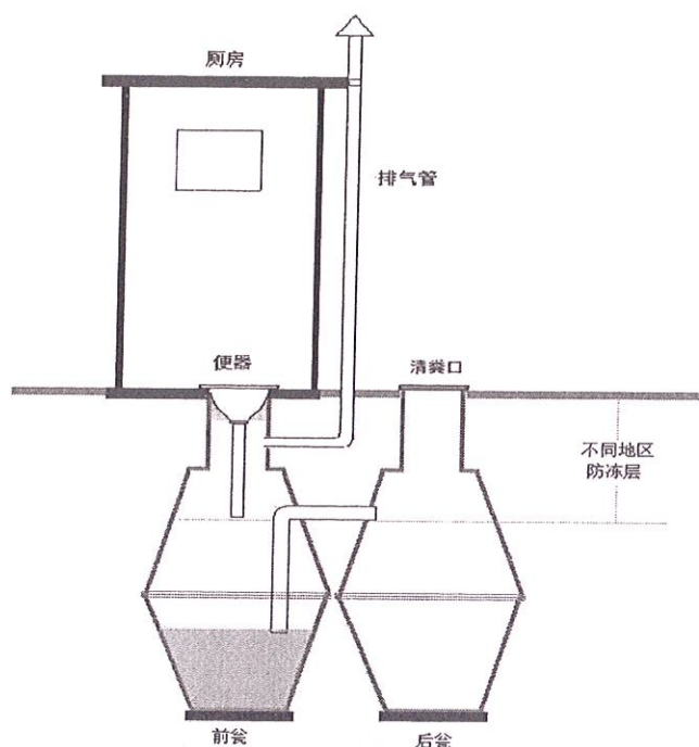
图 5.6-3 北方地区双瓮式户厕结构示意图
