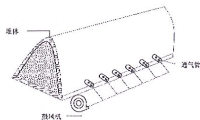
图 A.2-2 通气静态堆肥示意图
