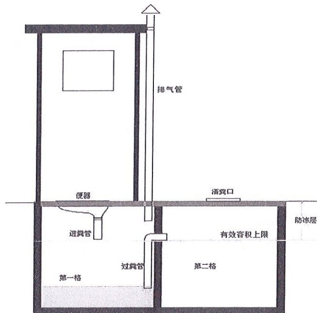
图 5.6-2 双格式户厕结构示意图
