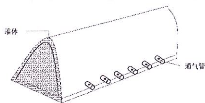
图 A.2-1 被动通气堆肥示意图
