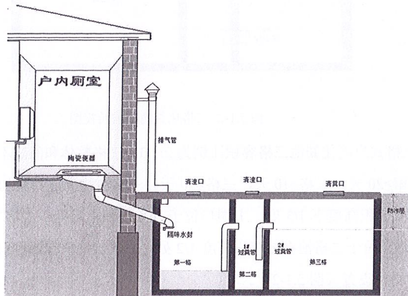
图 5.1-4 附建式三格化粪池式户厕示意图
