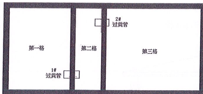
图 5.1-2 三格化粪池结构俯视图
