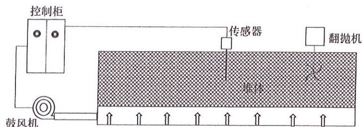
图 A.2-3 槽式堆肥示意图
