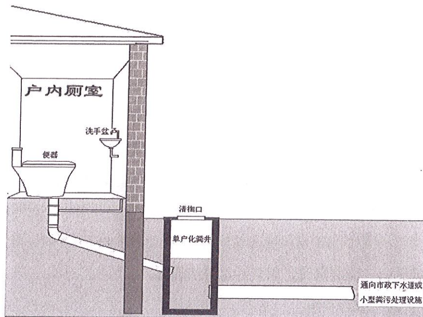
图 5.5-1 下水道水冲式户厕示意图
